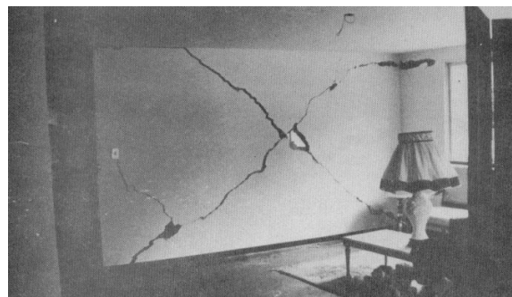
Daño tipo en paredes NS Comisión Presidencial, 1978b
