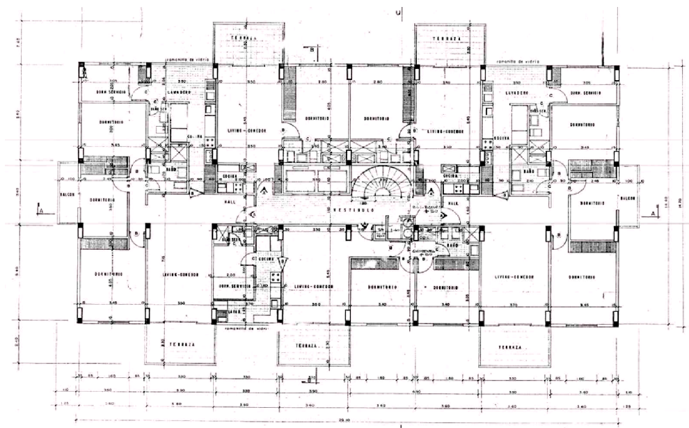
Planta tipo de Estructura y Arquitectura: Alcaldía de Chacao. Dirección de Ingeniería Municipal. Archivo.
